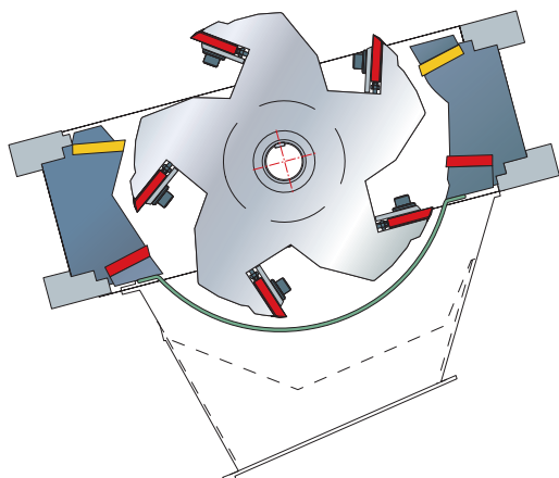
Rotor ouvert à 5 pales, universel.
