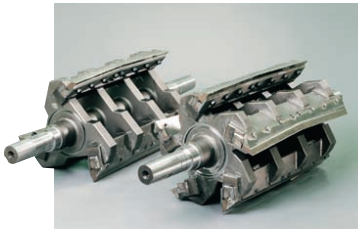
Rotors ouverts à 3 et 5 aubes.
