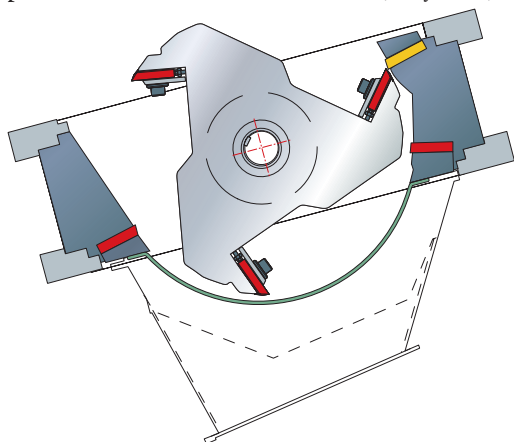
Rotor ouvert à 3 pales pour pièces volumineuses.
