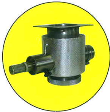
Pot d'aspiration en standard, possibilité 2 sorties
